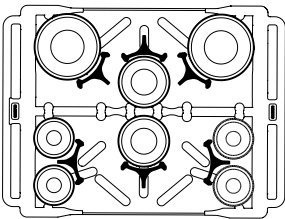
2列: 18.4 - 23.5 cm (每列 60 个盘子) 2列: 14.6 - 18.4 cm (每列 45 个盘子) 5列: 12.6 cm (每列 45 个盘子) 总容量: 390 (个盘子)
