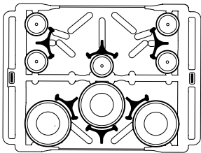
3列: 18.4 - 23.5 cm (每列 60 个盘子) 5列: 11.75 cm (每列 45 个盘子) 总容量: 405 (个盘子)
