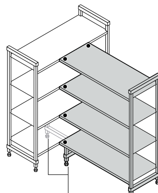
T型架 基础架 + 扩展架 每层搁板使用1套转角连接件，架体使用2个垫货支架。
