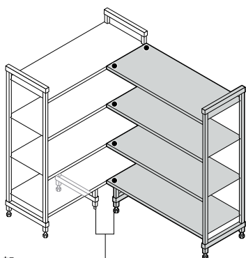
转角架 基础架 + 扩展架 每层搁板使用1套转角连接件，架体使用2个垫货支架。
