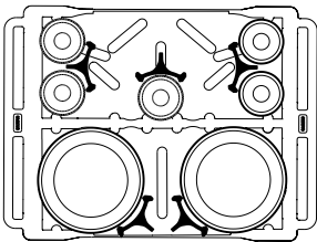
2列: 23.5 - 33 cm (每列 60 个盘子) 6列: 12.6 cm (每列 45 个盘子) 总容量: 345 (个盘子)
