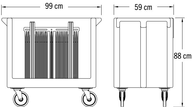
隔板可嵌入推车底部和后部的凹槽，以增加稳定性。
