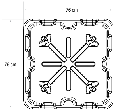
型号: ADCSC带有4个分隔柱
