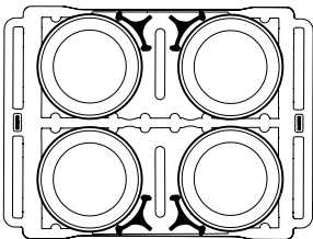
餐盘尺寸: 23.5 - 33 cm 4 列 (每列 60 个盘子) 总容量: 240 (个盘子)
