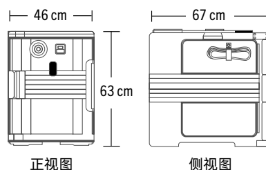
正视图
