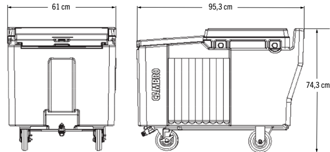
ICS175L (正面 / 宽度)
