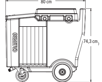
ICS125LB (Büyük, manevra tekerleğiyle birlikte)
