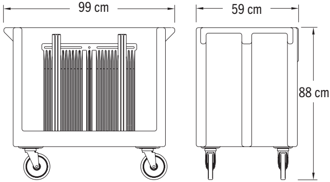
Seperatör, ek stabilite sağlamak için arabanın tabanına ve arka kısmına entegre edilmiş yivlere oturur.
