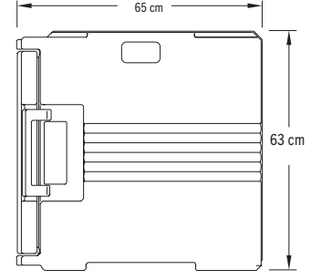
Yan Görünüm UPC400
