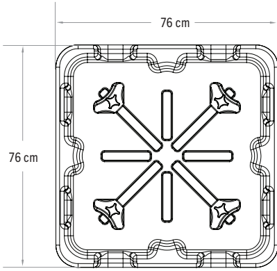
Model: ADCRC 4 sütunlu
