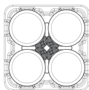
型号: ADCRC带有4个分隔柱
