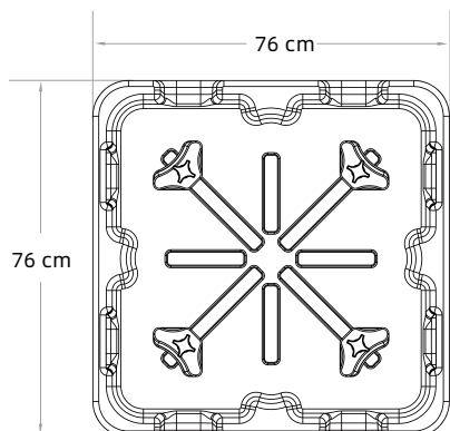
型号: ADCRC带有4个分隔柱
