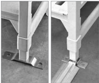
Bohrungsdurchmesser 0,95 cm.
