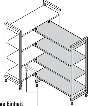
T-förmige Einheit Starteinheit + Anbaueinheitenseinheit mit 1 Satz Eckverbindern pro Regalboden und 2 Sockelgestellen.
