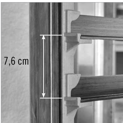
SCHIENENABSTAND Breiter 7,6 cm Schienenabstand bietet höchste Vielseitigkeit und Bedienkomfort.
