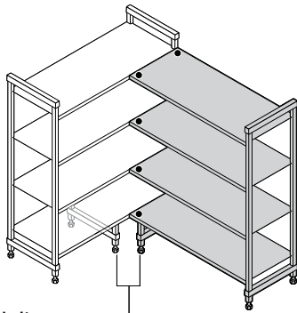
Eckeinheit Starteinheit + Anbaueinheitenseinheit mit 1 Satz Eckverbindern pro Regalboden und 2 Sockelgestellen.
