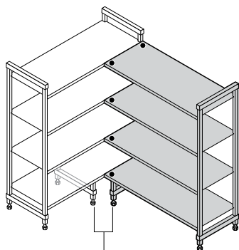
base + unidad adicional usando 1 juego de conectores de esquina por estante y 2 soportes de estiba.
