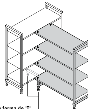
Unidad base + unidad adicional usando 1 juego de conectores de esquina por estante y 2 soportes de estiba.
