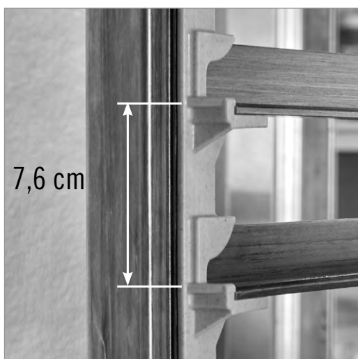
レール間隔 幅広7.6 cmのレール間隔で、最大 限の汎用性と使いやすさを実現。
