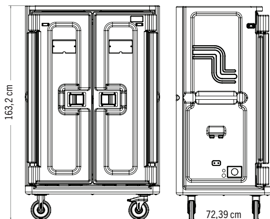
Frontansicht
